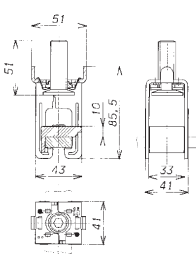
Morsetto 01759 - 01759 terminal
