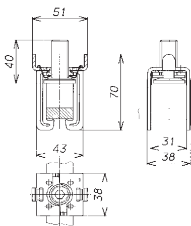
Morsetto 01319 - 01319 terminal
